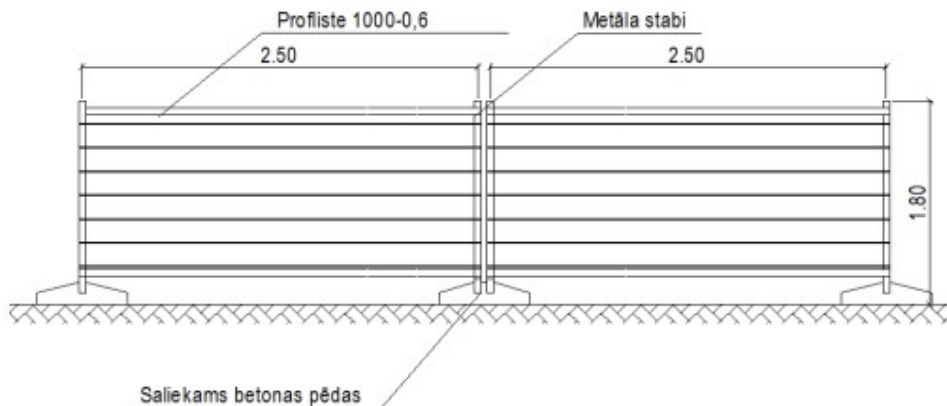
Attēls Nr.1. Mobilā pagaidu nožogojuma shēma.
